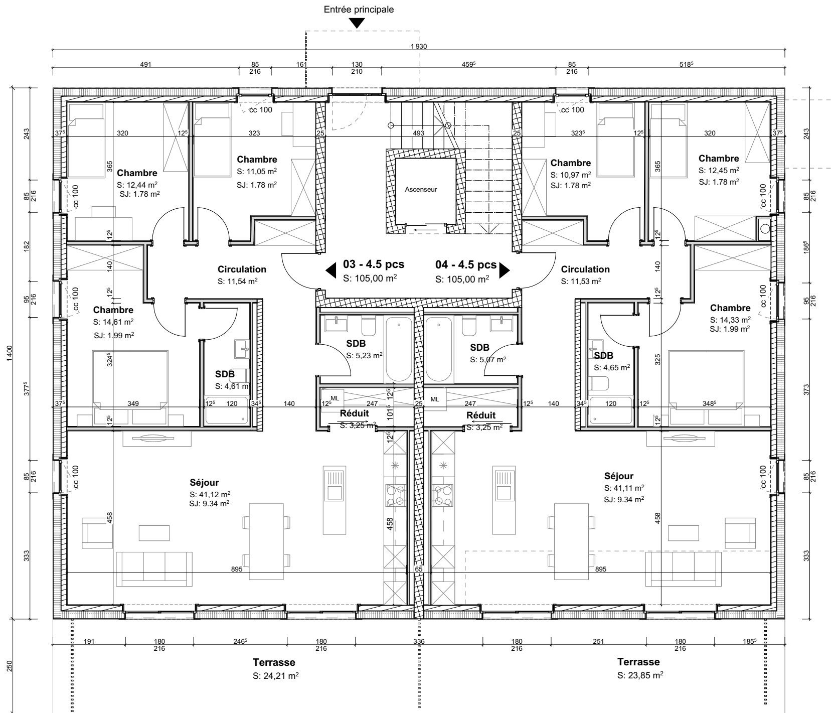
Plan du rez-de-chaussée_bât Est
