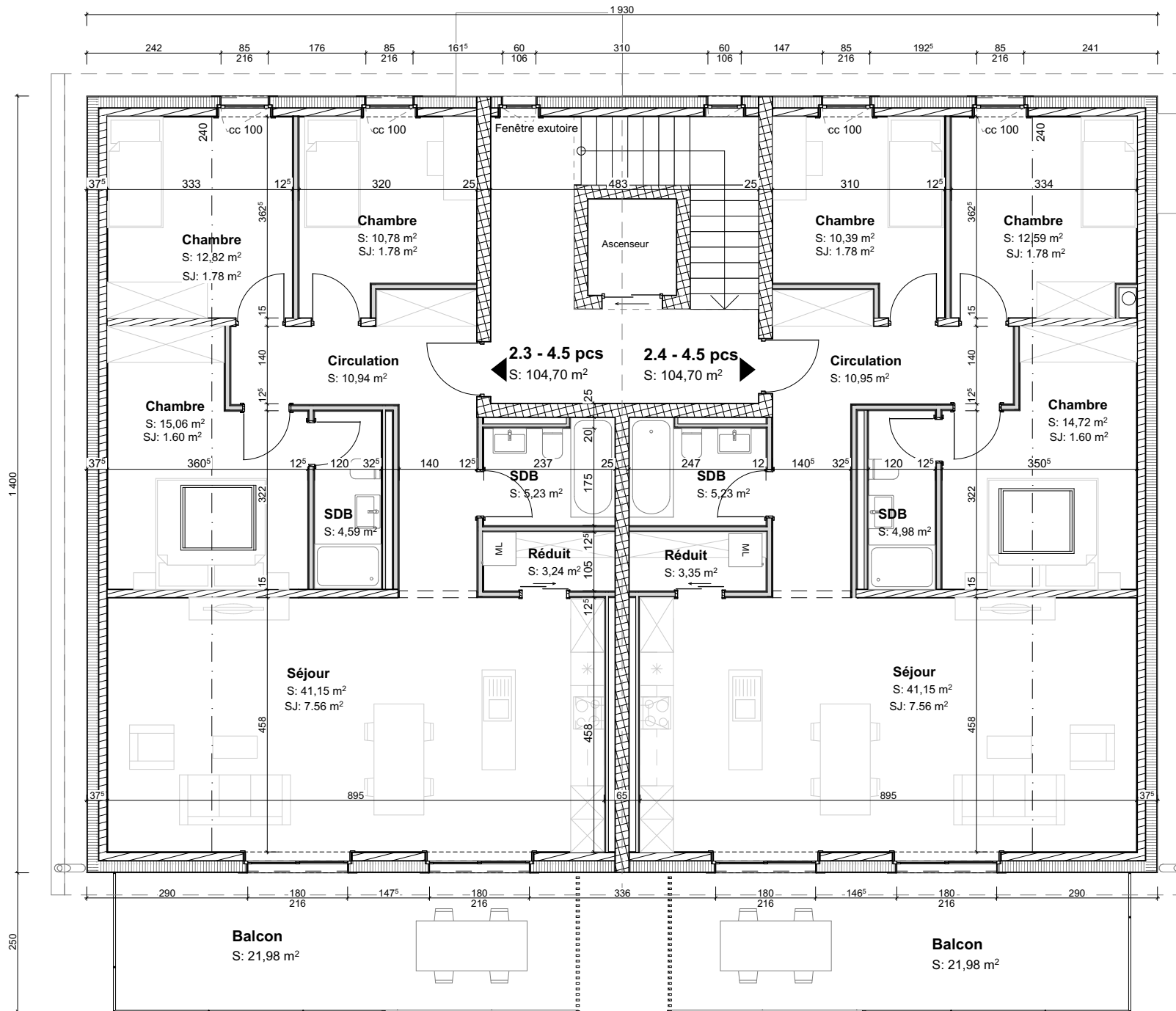
Plan des Combes _ bât Est
