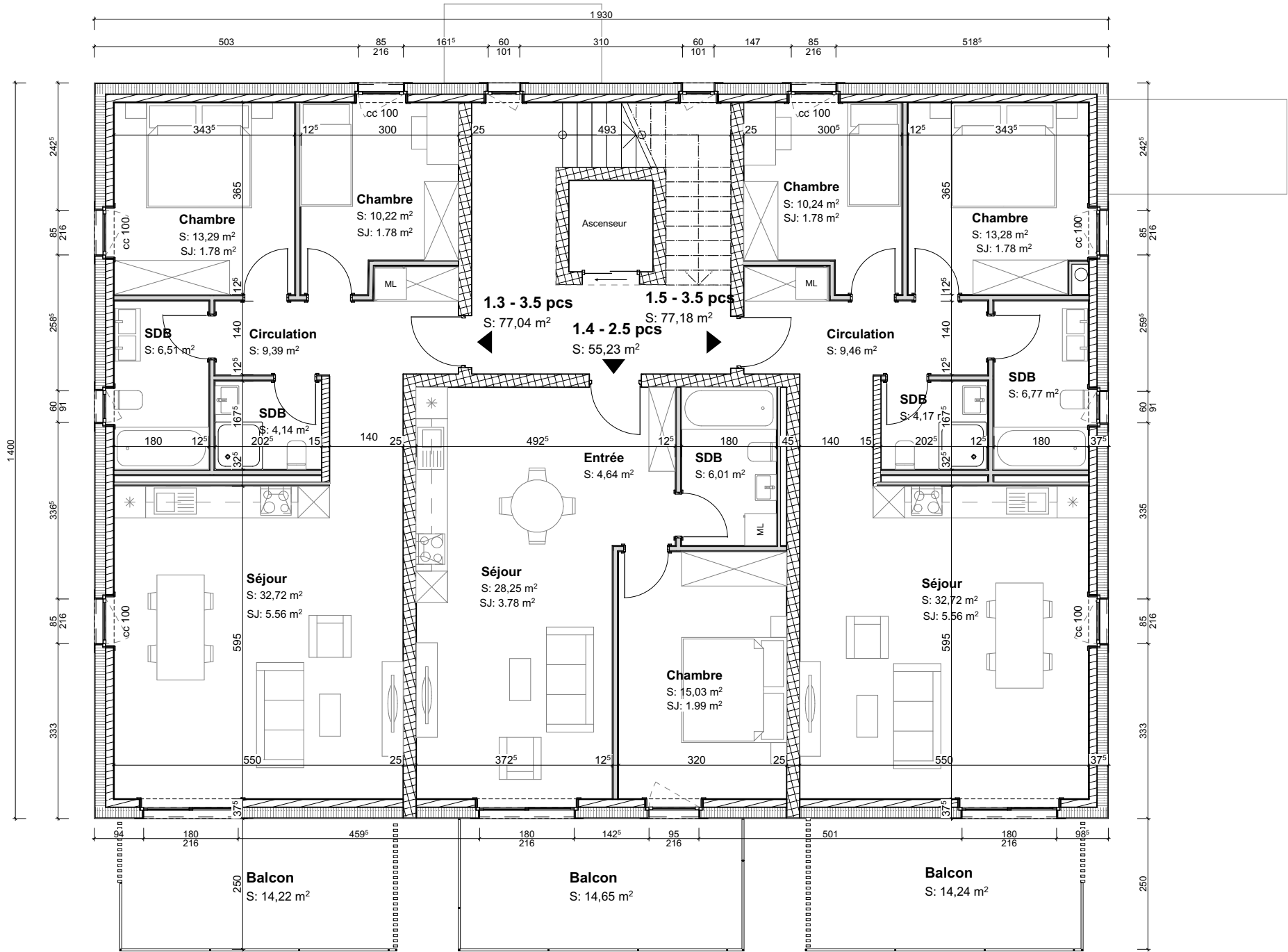
Plan Etage 1 _ bât Est
